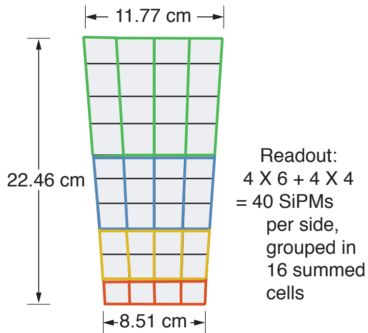
single module end (d)
